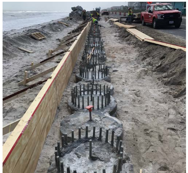
Küstenschutz mit 1.800 Bohrpfählen Flagler Beach, Florida, USA
