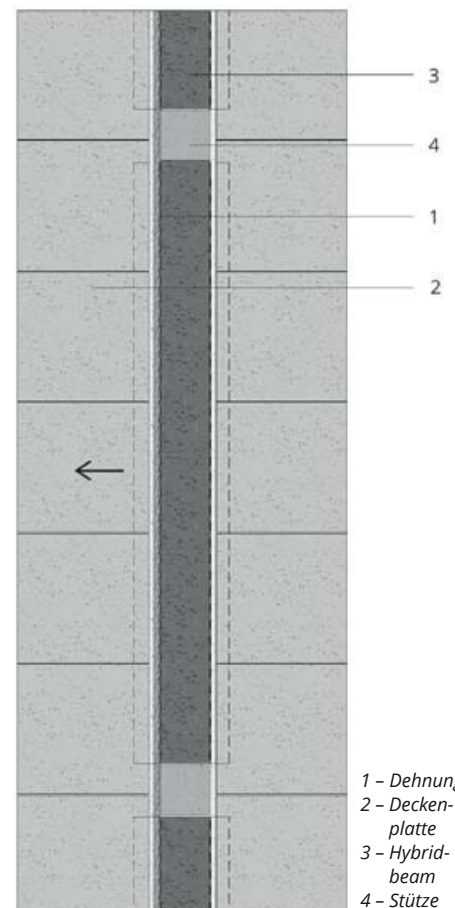
Decke mit Dehnungsfuge Grundriss
