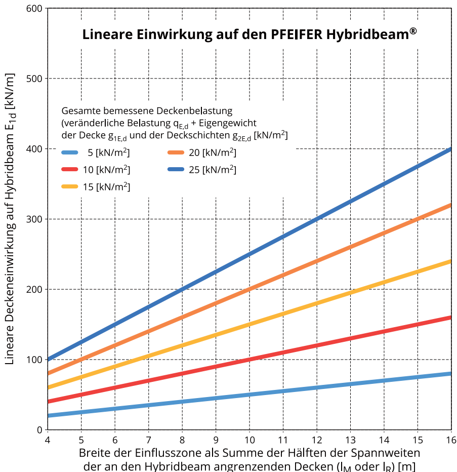
Eine Vorauswahl des statischen Deckensystems auf Basis von PFEIFER Hybridbeam® -Trägern mit den dafür notwendigen Parametern
