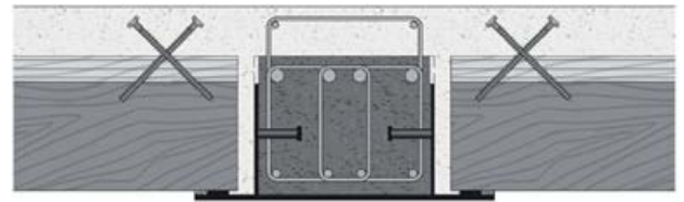
Holz-Beton-Verbunddecken (Ortbeton). Holzbalkendecke mit Deckel.
