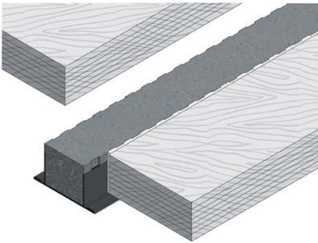
Holzdecken. Brettschichtholz.
