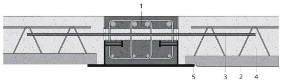
Hybridträger in Kombination mit einer einfeldrigen monolithischen Decke auf Fertigteileplatten
