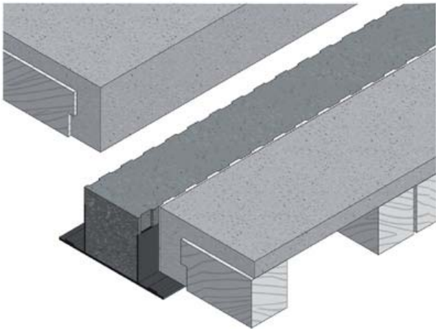
Holz-Beton-Verbunddecken (Betonfertigteil). Rippen aus Holz.
