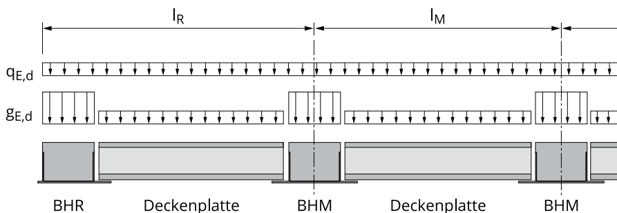
Eine Vorauswahl des statischen Deckensystems auf Basis von PFEIFER Hybridbeam® -Trägern mit den dafür notwendigen Parametern
