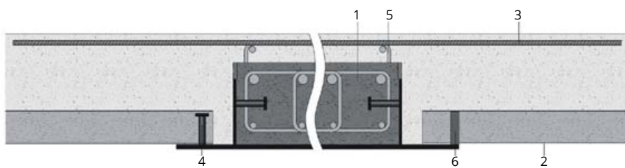
Hybridbeams für Verbunddeckenplatten auf Trapezblech mit geringerer Höhe als die Deckenplatte
