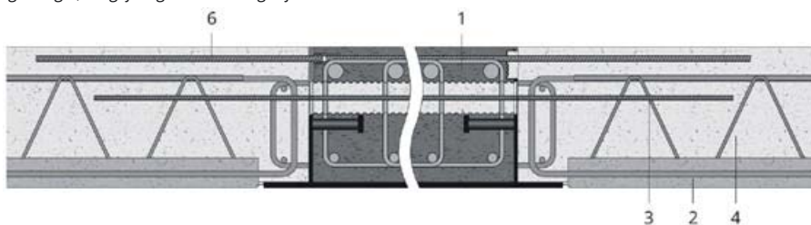
Abgehängte, vorgefertigte Plattenträger für Elementdecken
