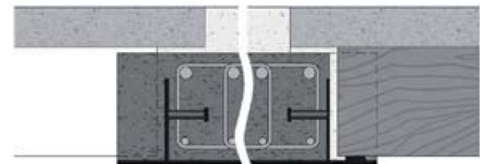
Holz-Beton-Verbunddecken (Betonfertigteil). Rippen aus Holz.
