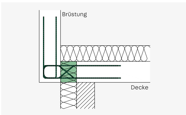
ISOPRO® 120 F - Einbausschnitt einer vorgesetzten Brüstung mit Wärmedämmverbundsystem
