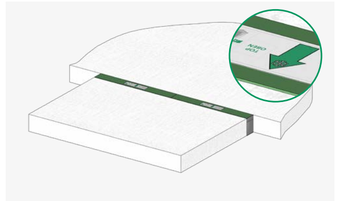
ISOPRO® 120 - Einbaurichtung
