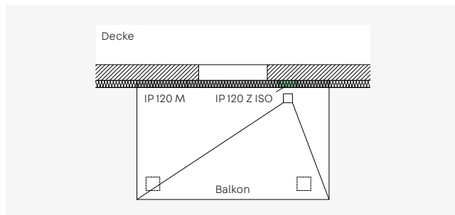
ISOPRO® 120 Z ISO - Balkon auf Stützen - Z ISO Elemente im Bereich der Entwässerung
