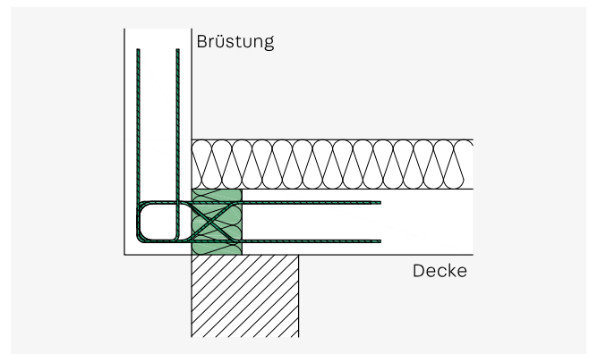
ISOPRO® 120 F - Einbausschnitt einer vorgesetzten Brüstung mit einschaligem Mauerwerk
