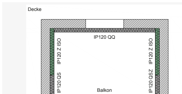
ISOPRO® 120 Z ISO - Loggia mit punktueller Lagerung
