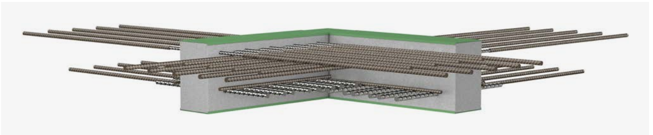
ISOPRO® 120 C – Ansicht Deckenseite
