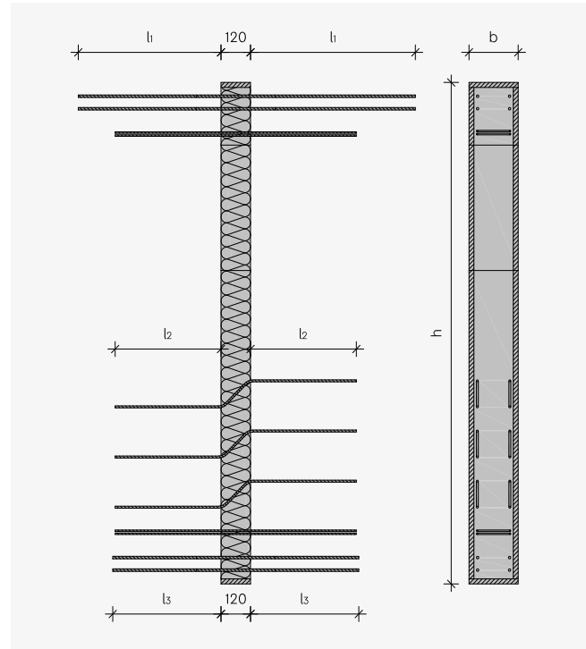
ISOPRO® 120 W R 90 - umlaufende Brandschutzplatten
